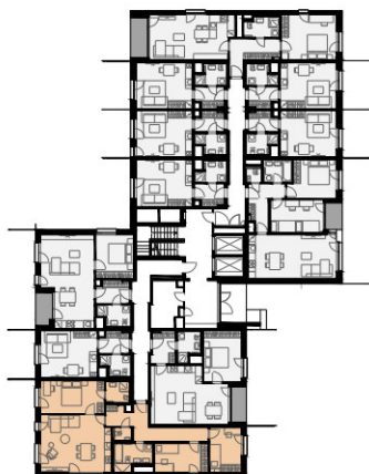
PŮDORYS PATRA
